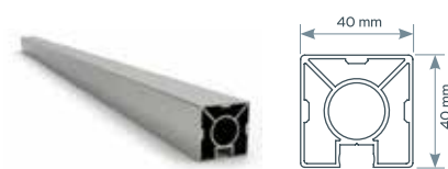
EX-3958833716 Κολόνα 40x40 mm με αυλάκι - 1145 gr Column 40x40 mm with channel - 1145 gr
