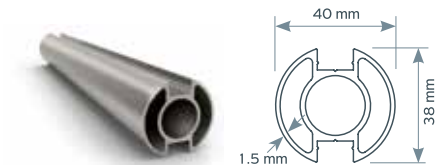
EX-3955456616 Κολόνα Ø40 Ελαφριά 1.5mm - 971 gr Column 40 mm Light 1.5mm - 971 gr
